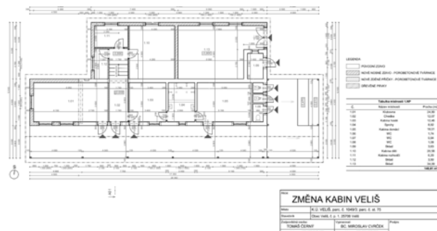
Změna kabin Veliš – půdorys 1. NP
